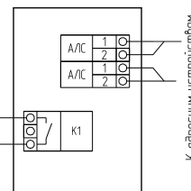
Рисунок 3- Модуль релейный РМ-1C прот. R3
